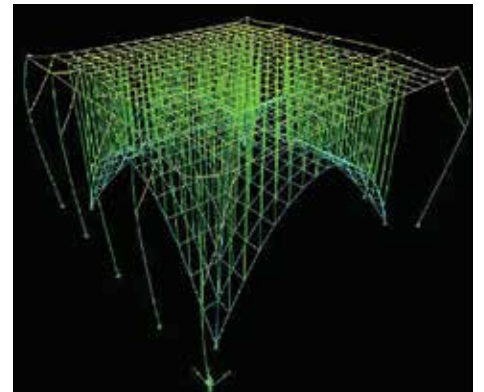
Figura 2: Observación y corrección de deformaciones estructurales del sistema propuesto.
